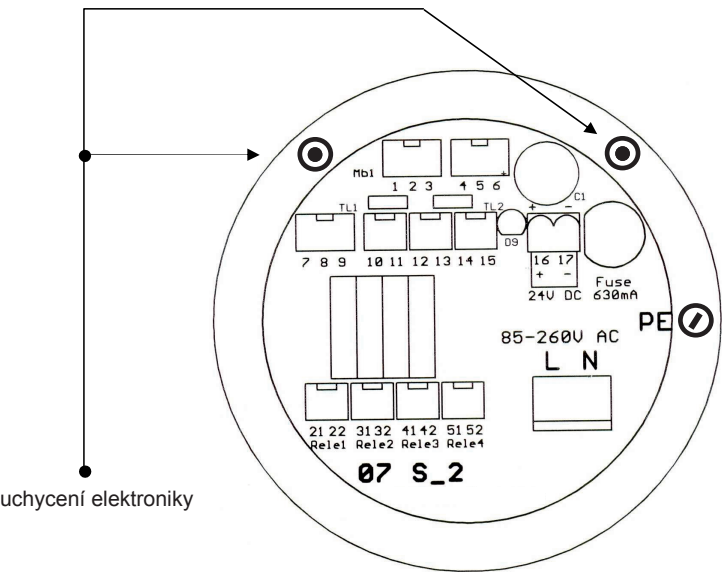
Rozmístění svorkovnic
